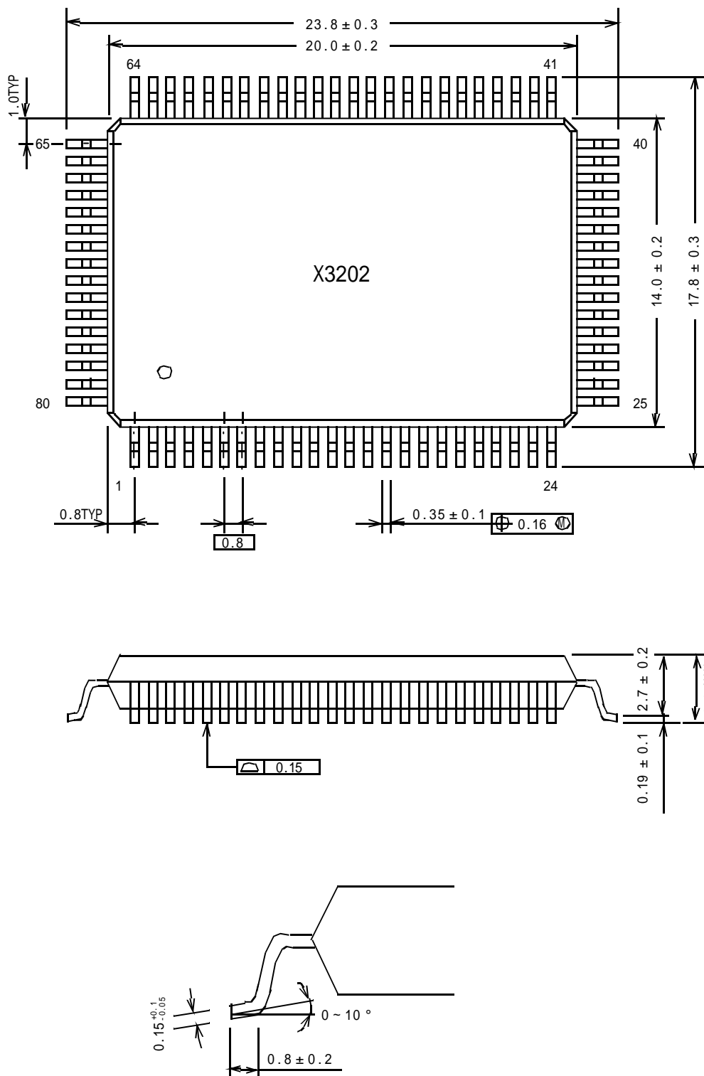
図 1-2: パッケージ寸法
