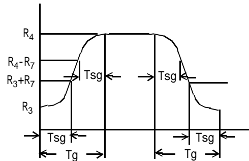
図 5-1: S字加減速
