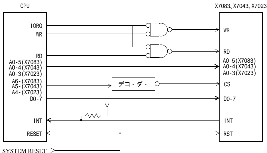
図 1-8: Z80 とのインターフェース例
