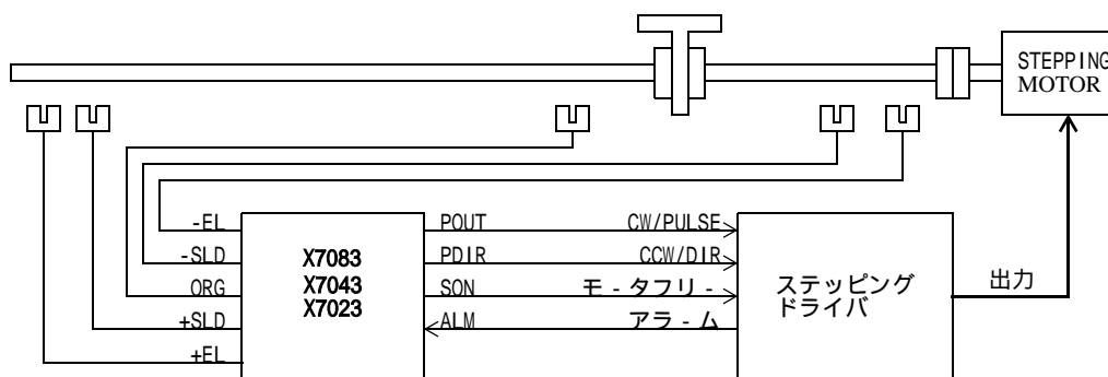
図 1-7: ステッピングモータインターフェース例
