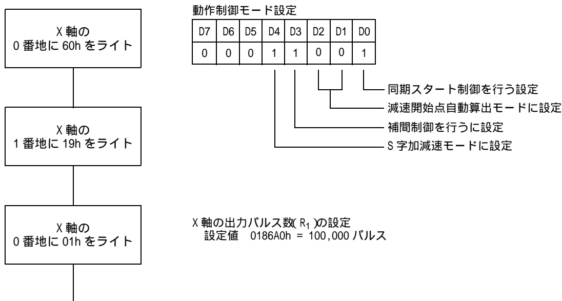
図 10-8: 直線補間駆動のフローチャート (X 軸、Y 軸の場合)
