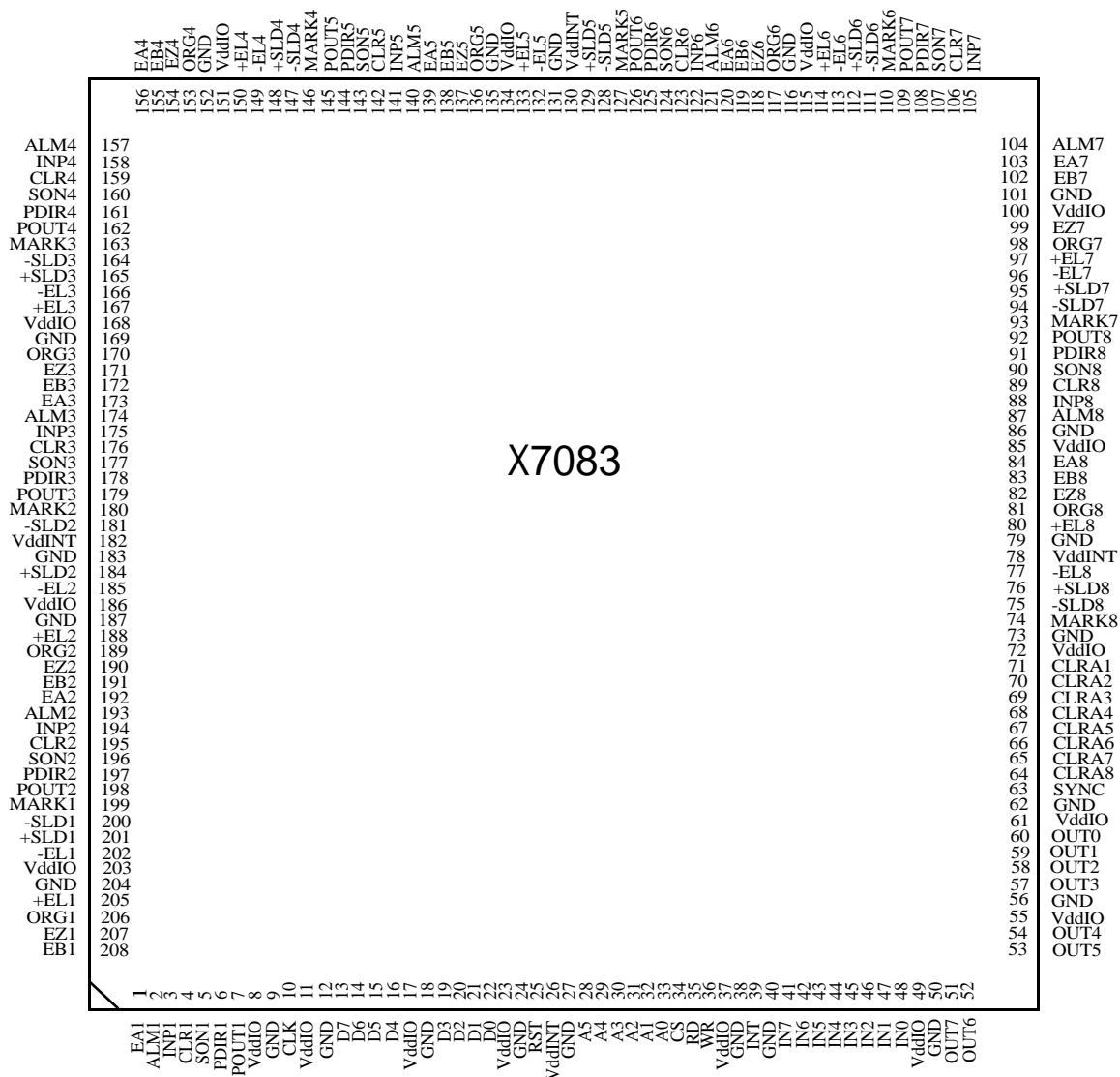
図 1-5: ピン配置図
