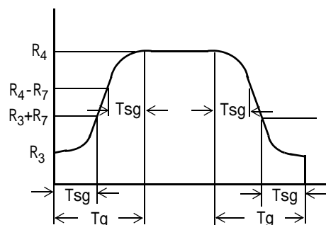
図 5-1: S字加減速の状態
