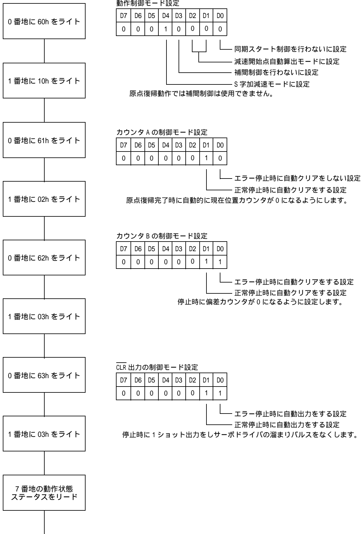
図 10-6: 原点復帰のフローチャート (#1 軸の場合)
