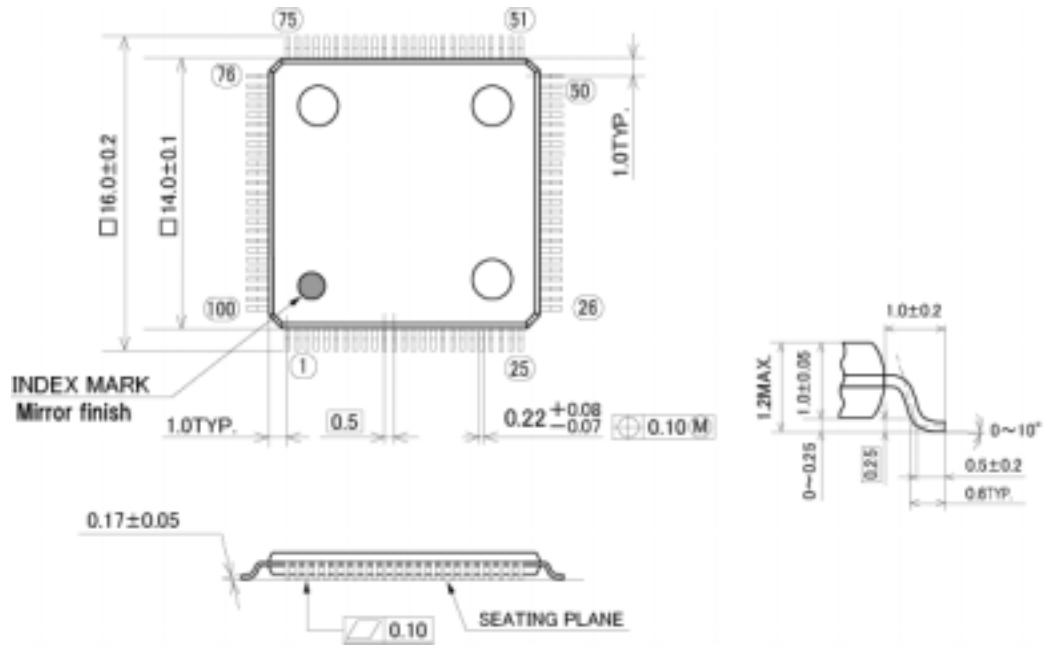
図 1-4: パッケージ寸法図 (X7023)
