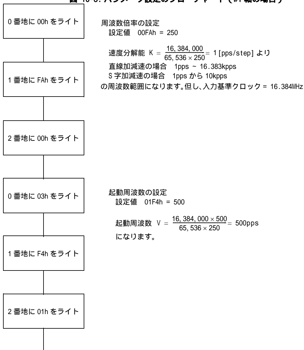
図 10-3: パラメータ設定のフローチャート (#1 軸の場合)
