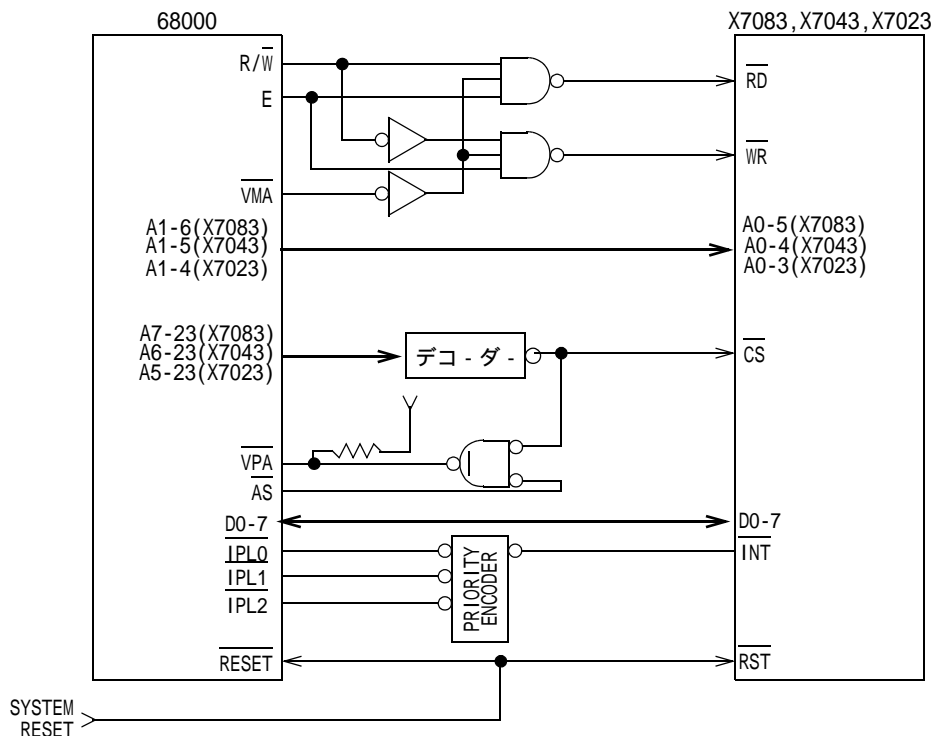
図 1-9: 68000 とのインターフェース例
