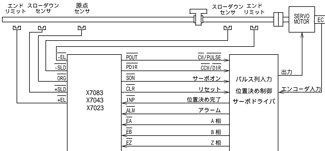
図 1-6: サーボモータインターフェース例
